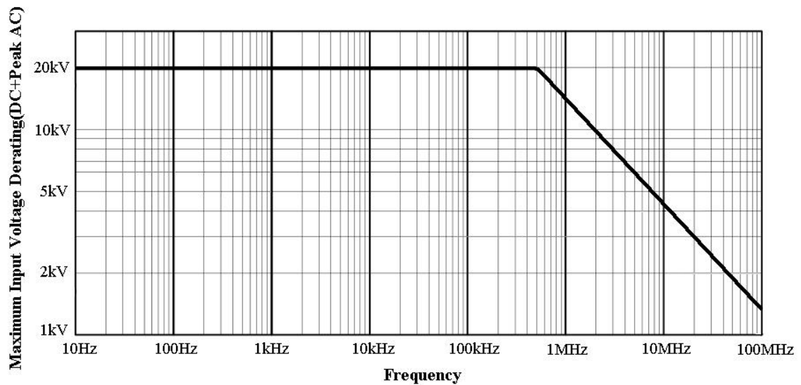
图 1：最大输入电压 VS 频率曲线
