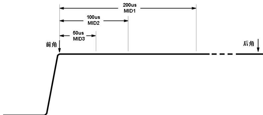
图 2: 补偿区域示意图
